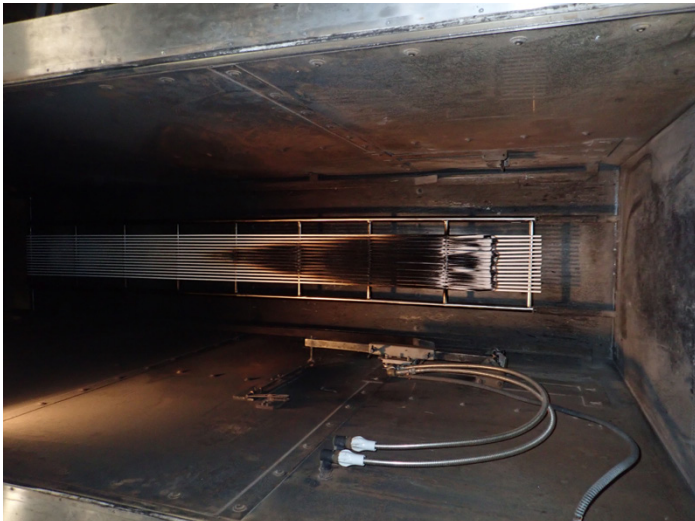
Bild 2: Messung der Wärmefreisetzung und Raucherzeugung von Kabeln nach EN 50399 – nach dem Versuch (Quelle: VDE Prüf- und Zertifizierungsinstitut GmbH)
