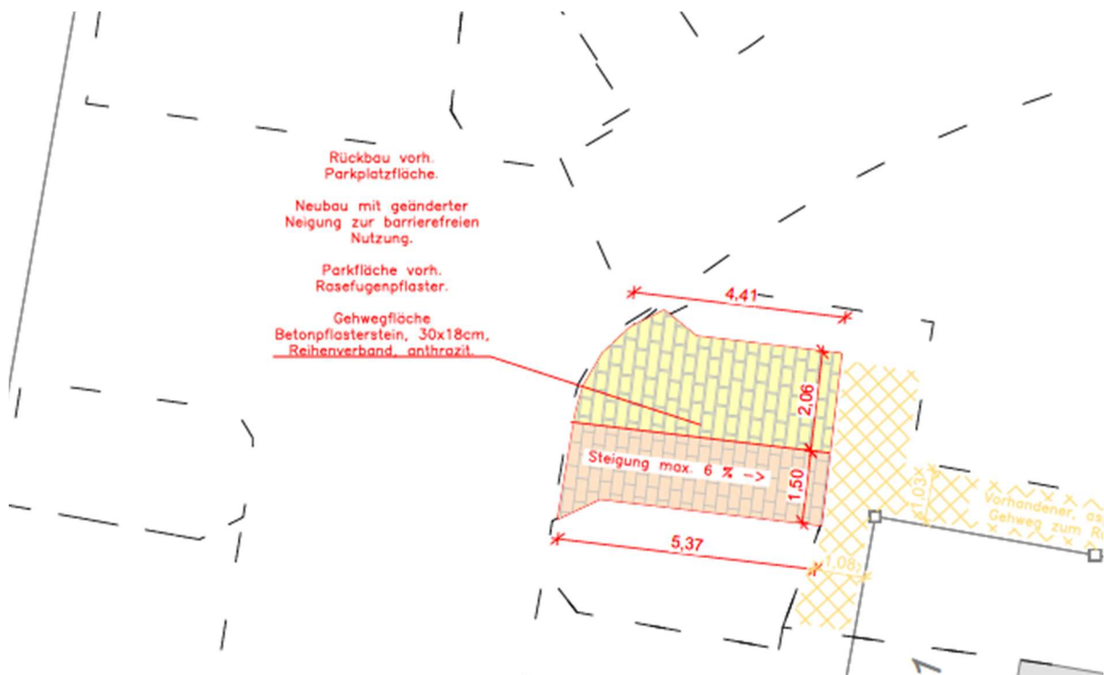
Entwurf zur Umgestaltung des personenbezogenen Parkplatzes
