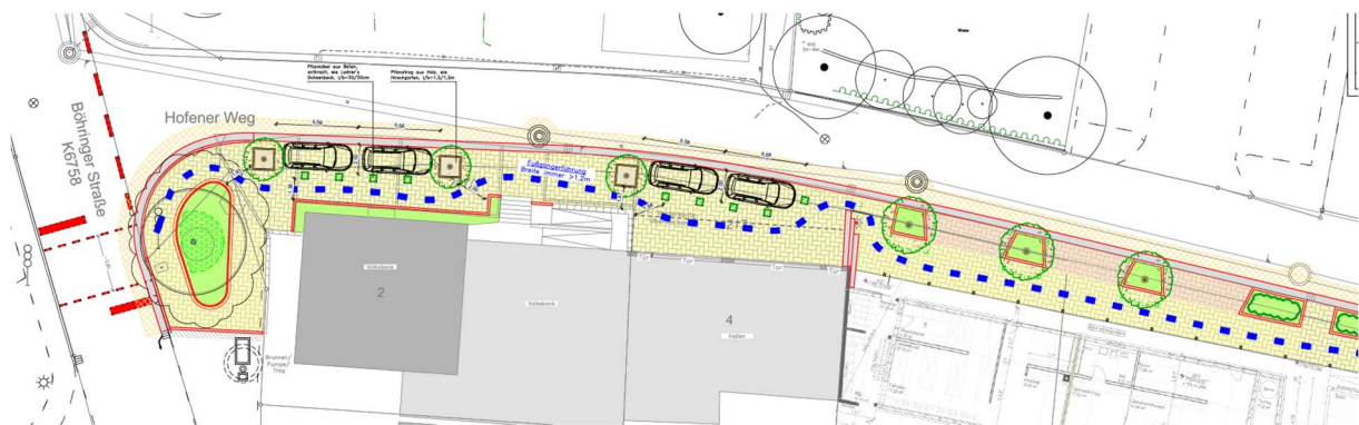
Bild 2 Entwurf der Gesamtplanung
