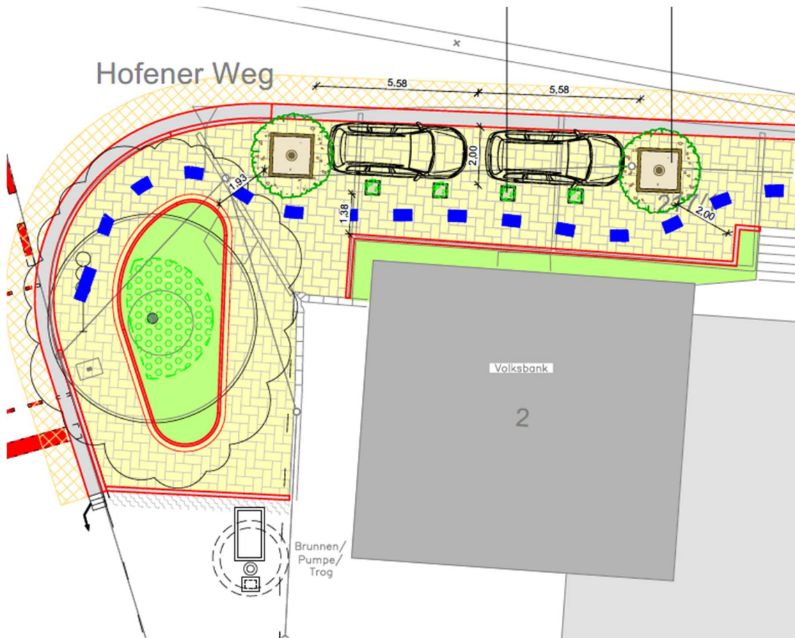
Bild 1: Entwurf der Erweiterung des Baumfeldes sowie des barrierefreien Umbaus
